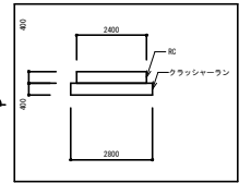
室外機用土台詳細 1/50
